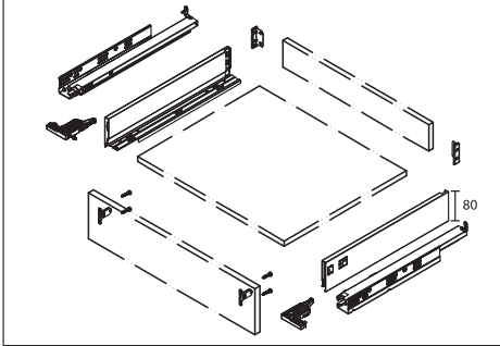
Componentes para cajón altura 80mm
