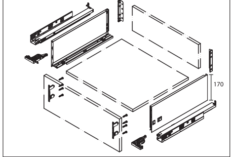
Componentes para cajón altura 170mm
