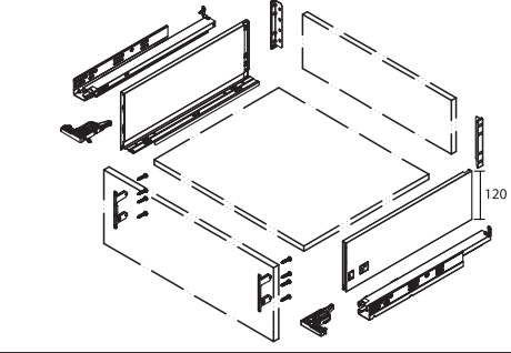
Componentes para cajón altura 120mm
